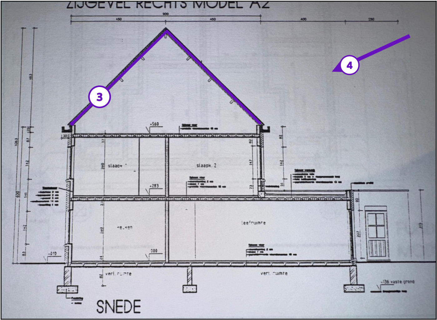
Legende van plan 1.4: Snede
