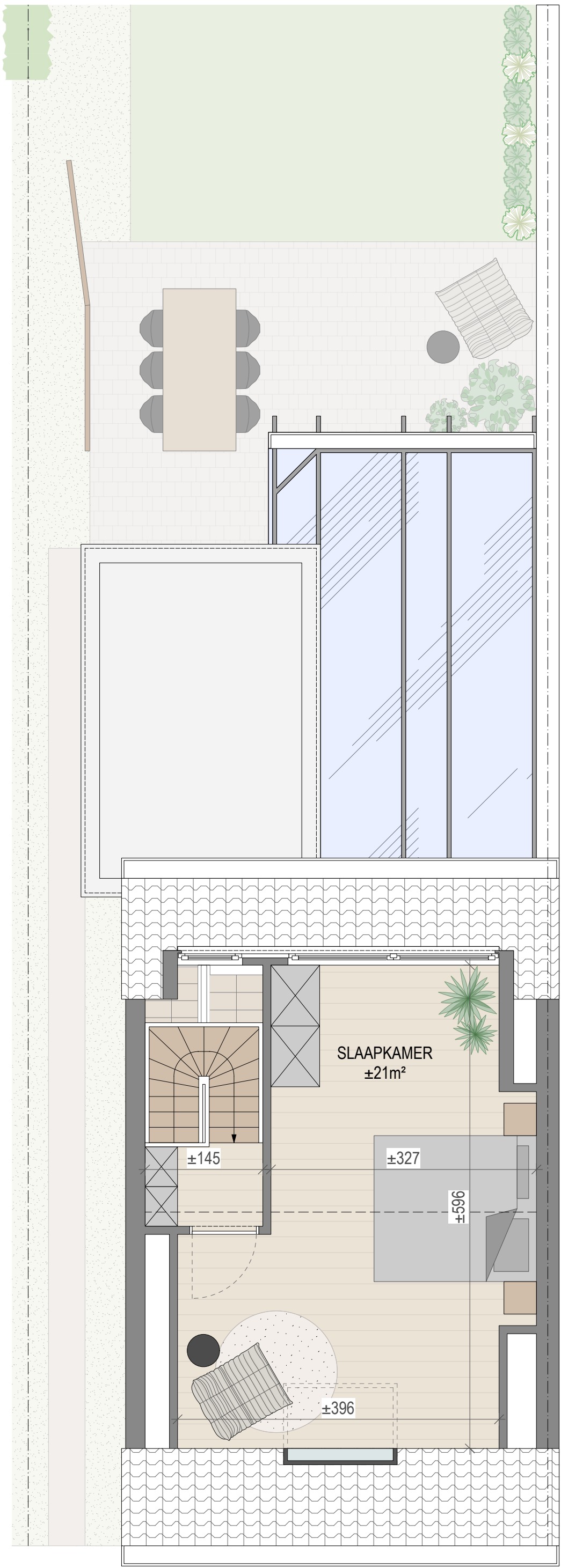
±520 TWEEDE VERDIEPING
