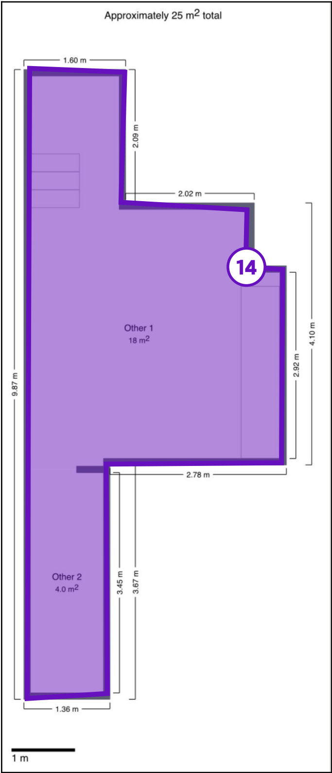
Legende van plan 1.3: Kelder kopie 2
