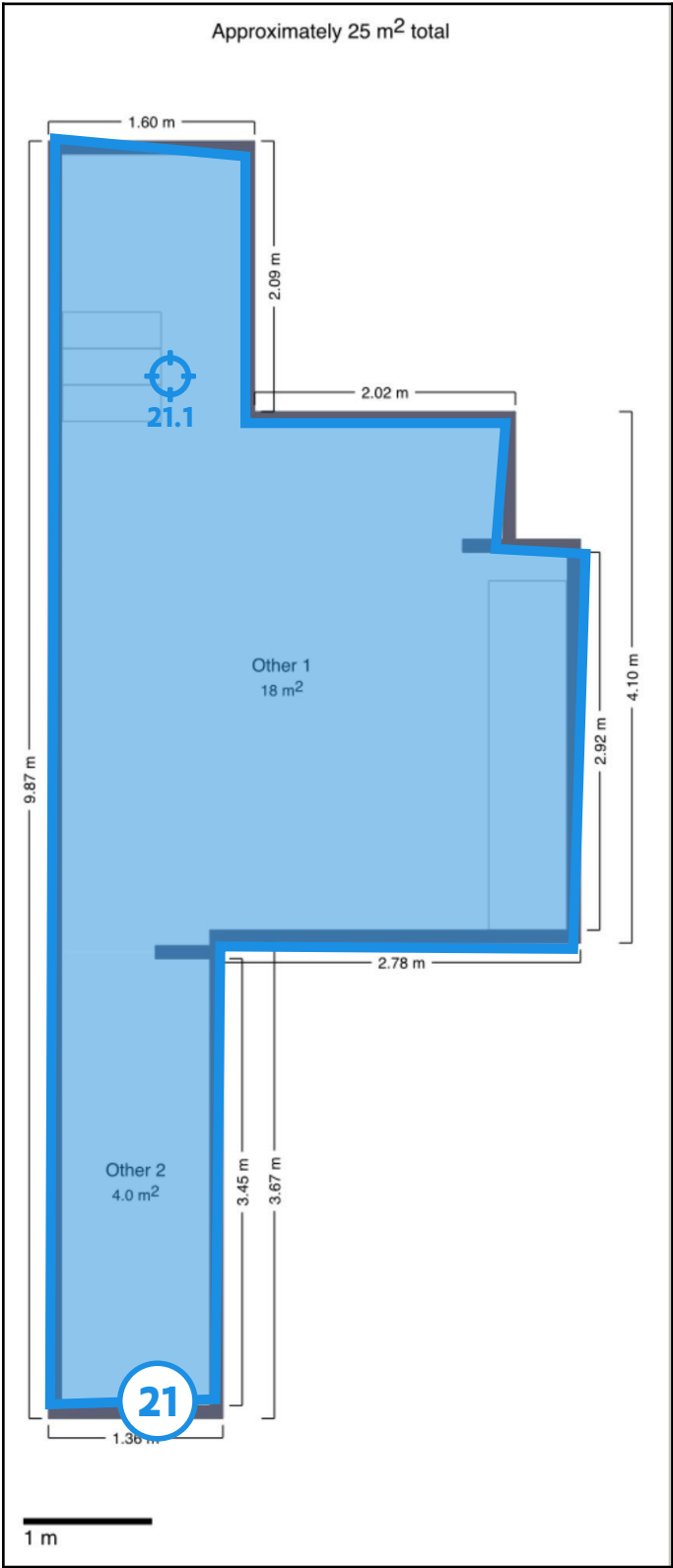
Legende van plan 1.2: Kelder kopie
