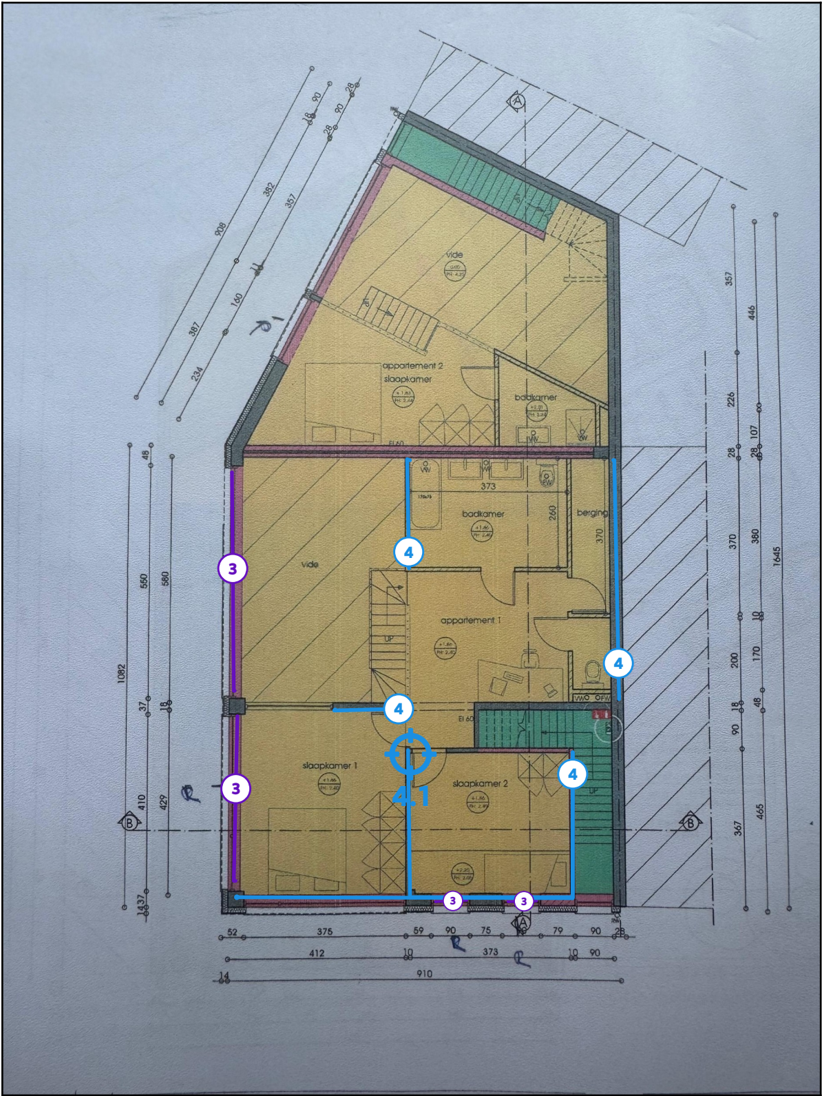
Legende van plan 1.2: Eerste verdieping
