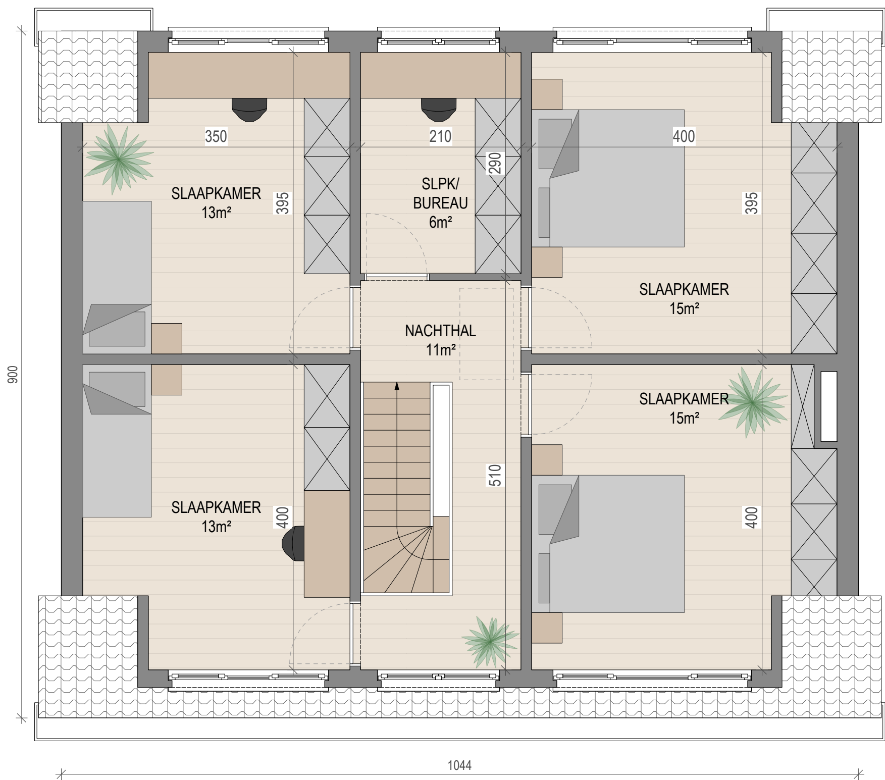
EERSTE VERDIEPING
