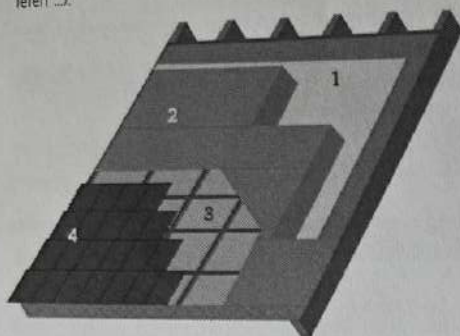
1. Dampscherm | 2. Isolatie | 3. Onderdak | 4. Dakbekleding
